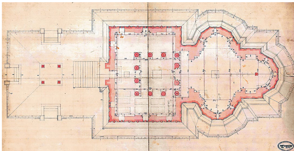
План Цркве Усијења Пресвете Бојородице према Лекомшћу ди Нуцу, крај XIX века
