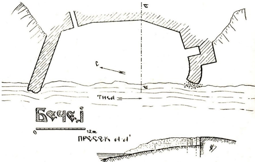
Пресек у тврђења на Тиси
